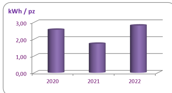
Figura5–Energiaconsumata/pzprodotti(dal2020al2022)
